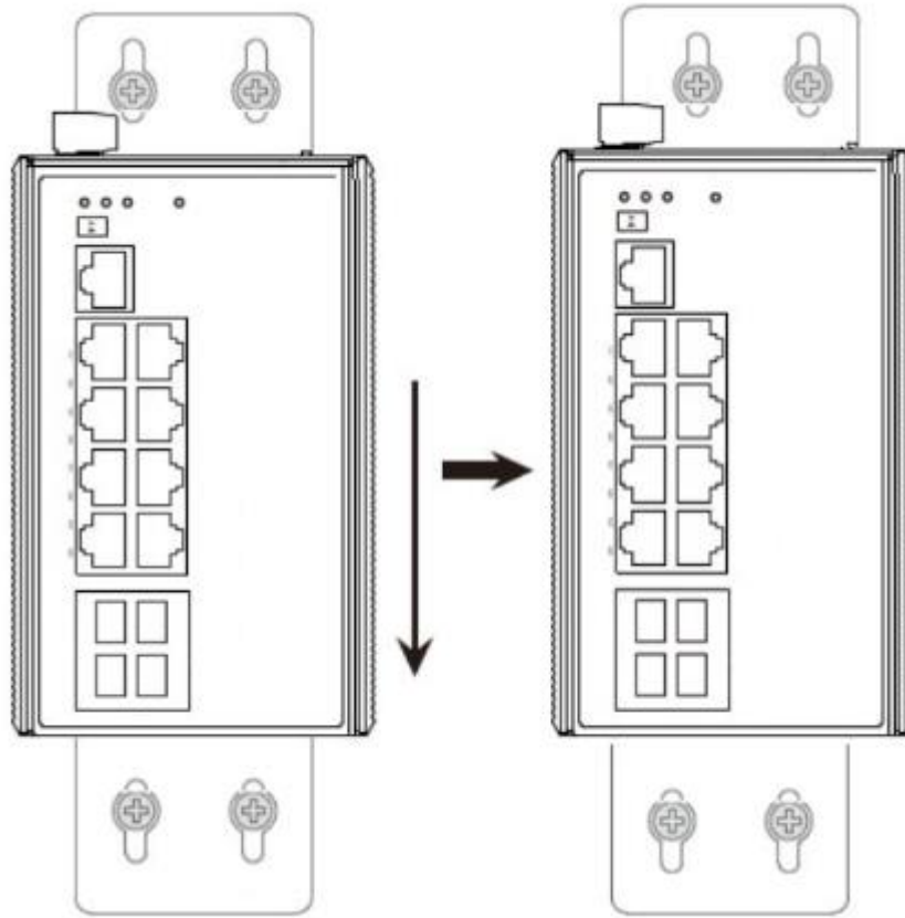
工业机壁挂式安装示意图
