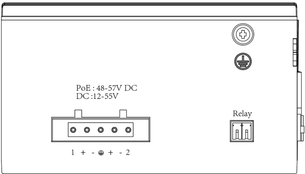
图 2-2 交换机侧面板示意图
