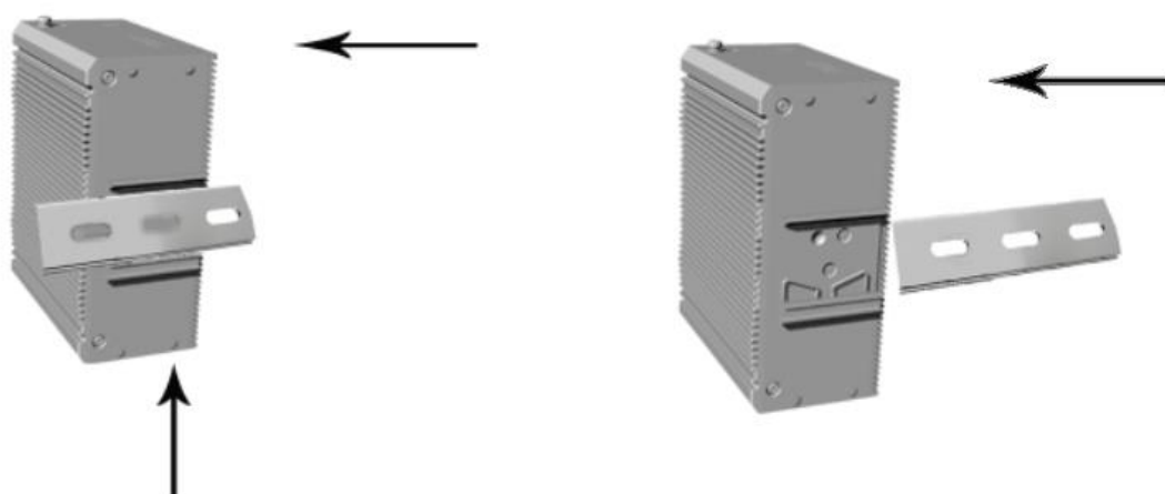
图 3-2 工业机导轨拆卸示意图
