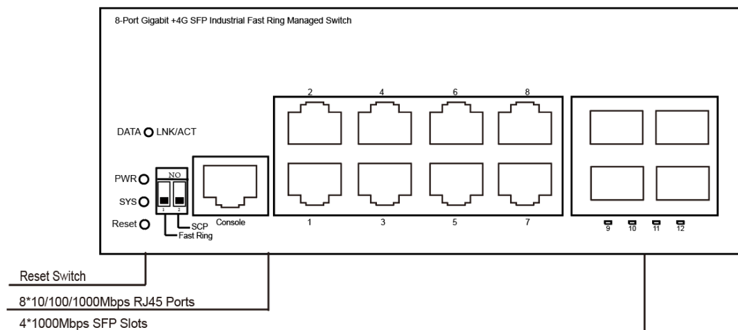
图 2-1 交换机前面板示意图
